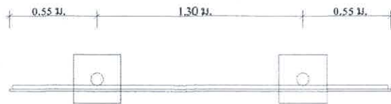
แปลน
